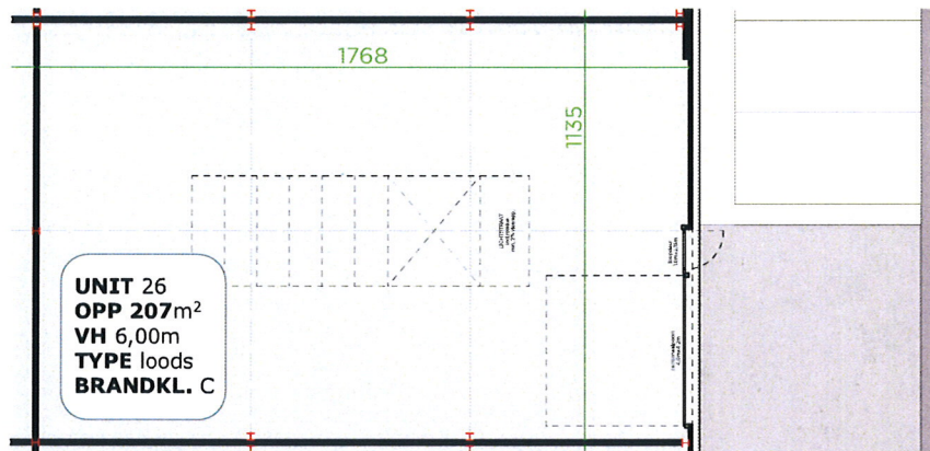
Grondplan
