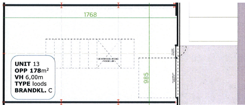
Grondplan
