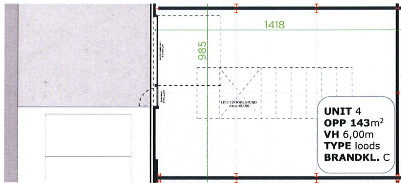
Grondplan
