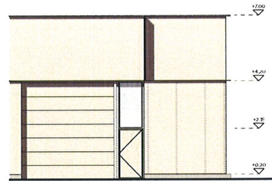
Voorgevel
