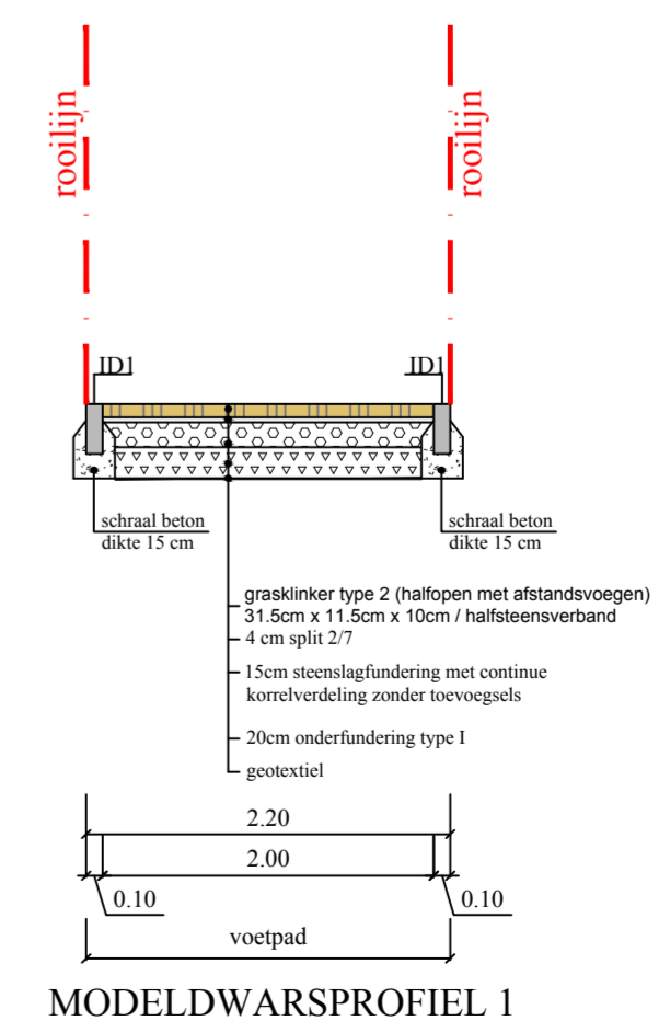
MODELDWARSPROFIEL 1
