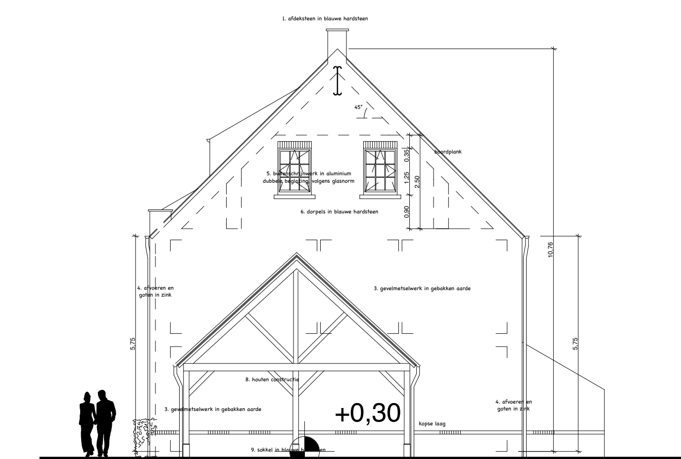
RECHTERZIJGEVEL - lot 5 schaal: 1/100
