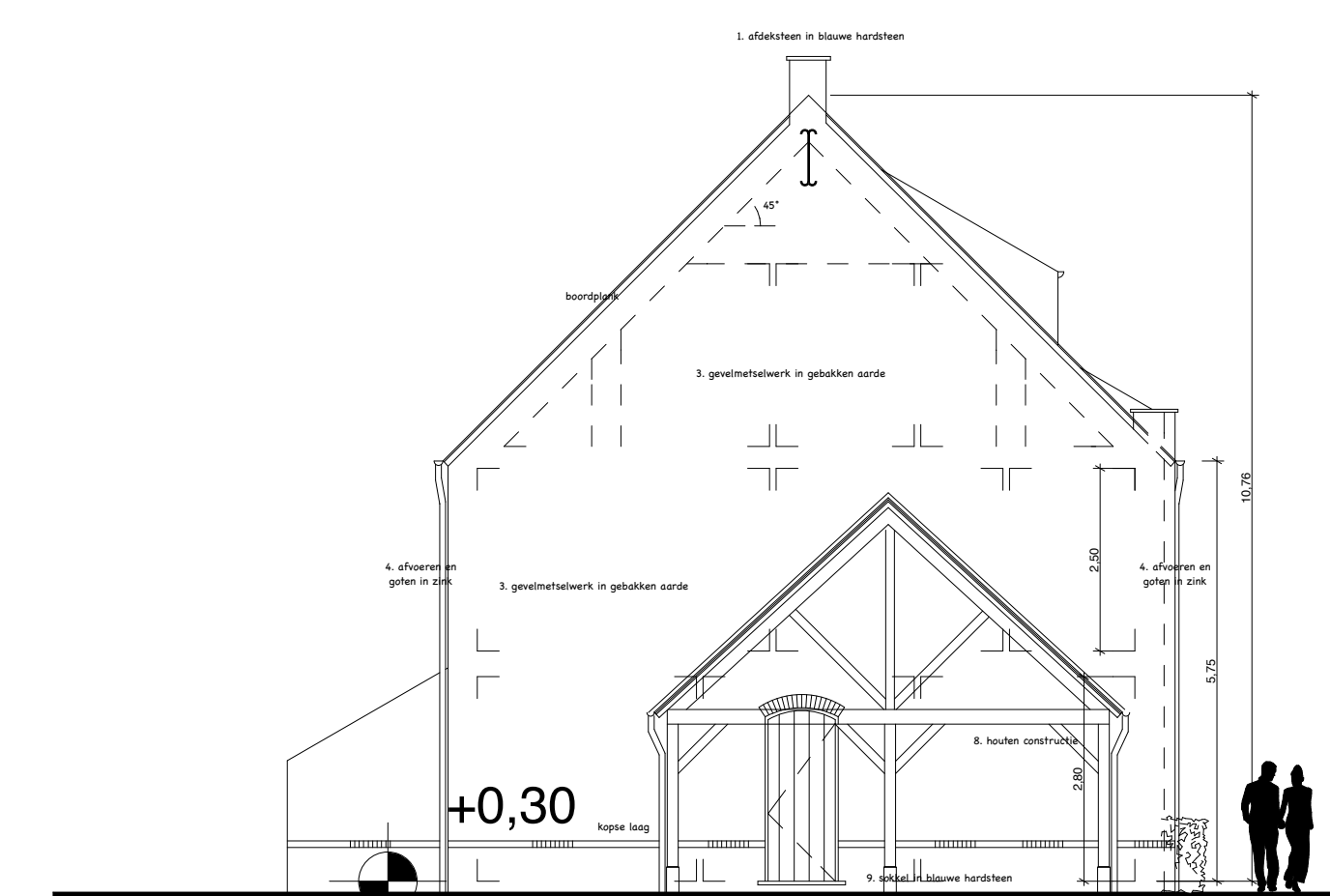
LINKERZIJGEVEL - lot 4 schaal: 1/100
