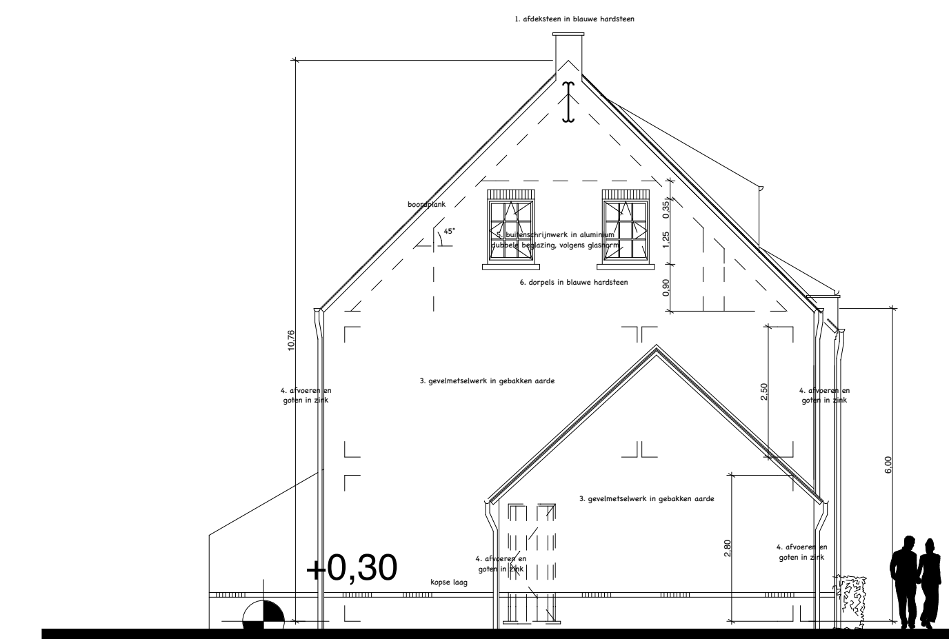
LINKERZIJGEVEL - lot 1 schaal: 1/100
