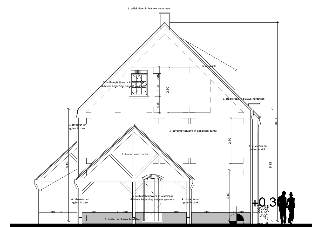
LINKERZIJGEVEL - lot 6 schaal: 1/100
