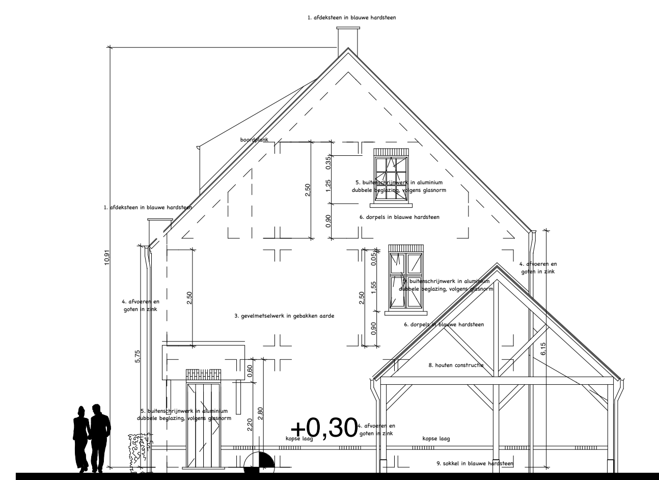
RECHTERZIJGEVEL - lot 8 schaal: 1/100
