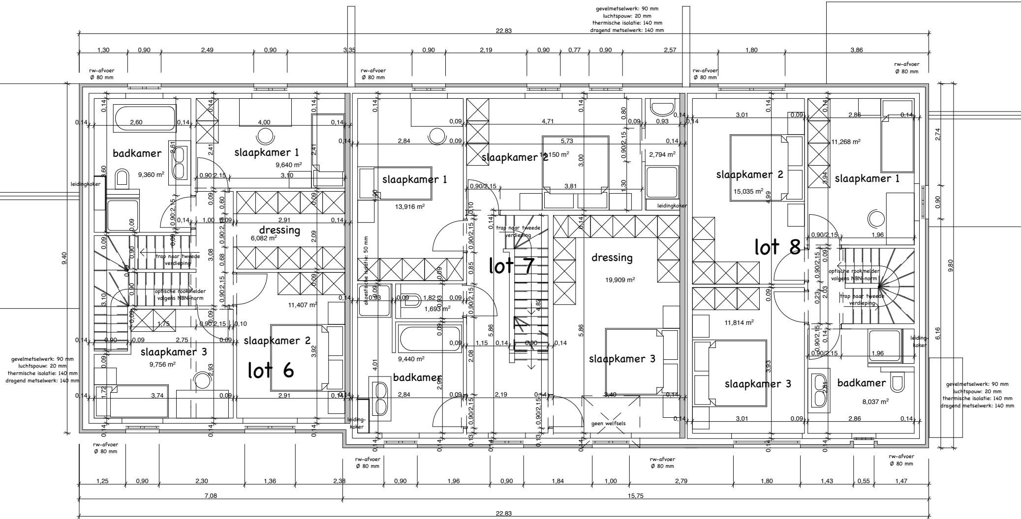
EERSTE VERDIEPING - lot 6 TEM 8 schaal: 1/100
