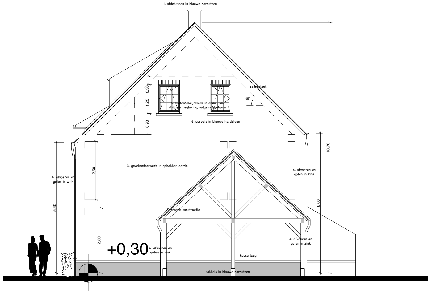
RECHTERZIJGEVEL - lot 3 schaal: 1/100
