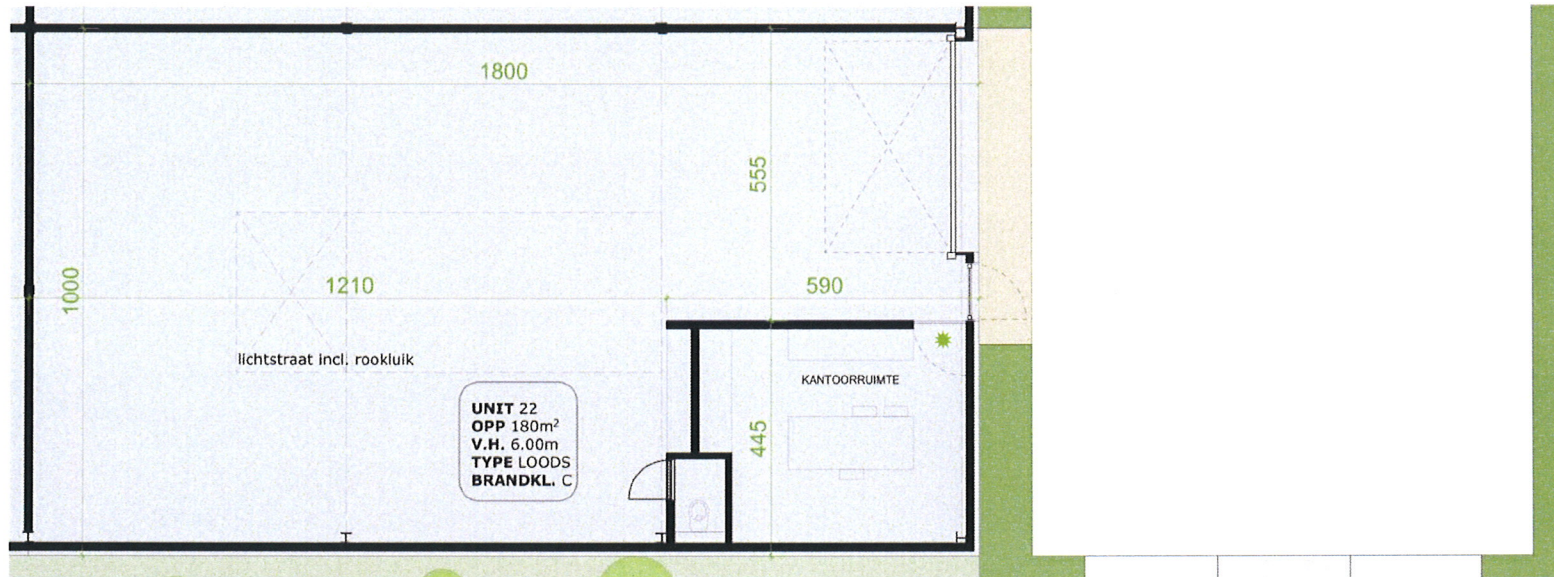
GRONDPLAN
