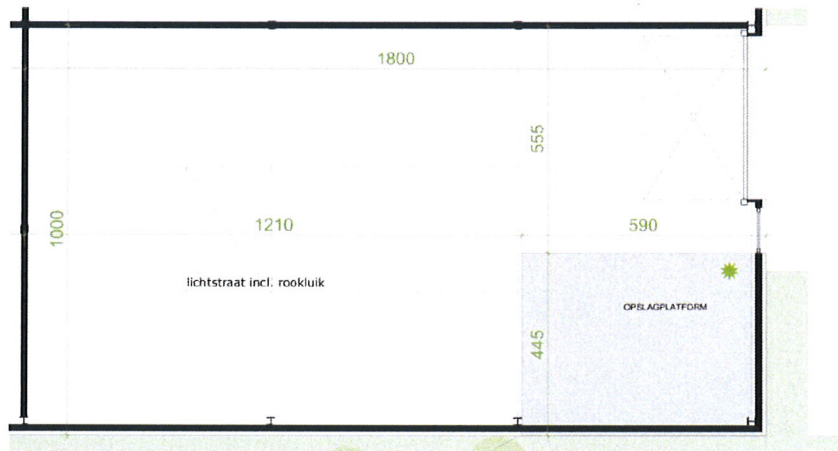
VERDIEPINGSPLAN
