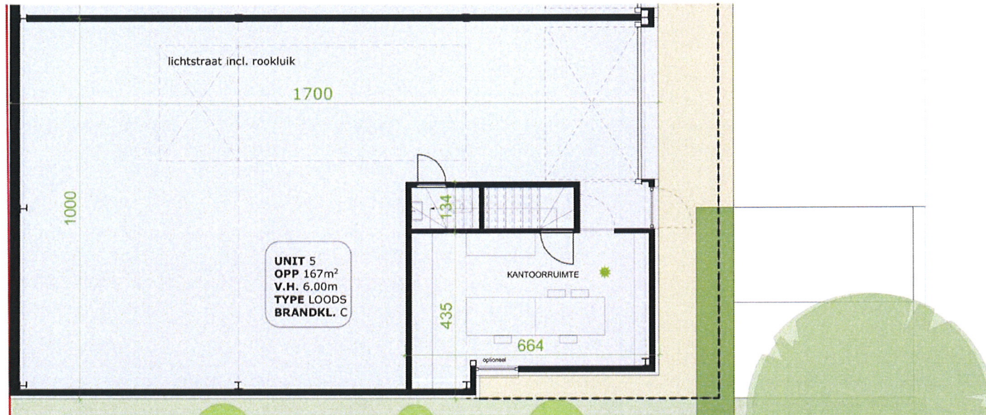
GRONDPLAN
